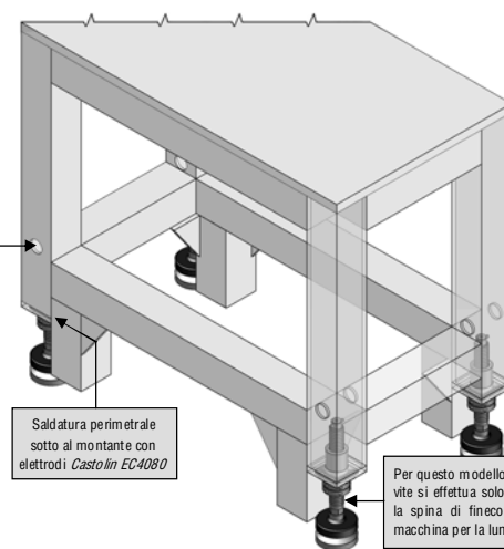
Rappresentazione indicativa di una base per macchina con l'utilizzo di Stabilizzatori livellanti art.SLV...RB+CFQ mod.RB...S2
