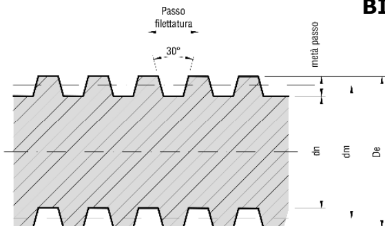
Filettatura trapezoidale a profilo "ISO"
