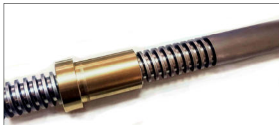
Esempio di accoppiamento chiocciola e barra filettata TR 50x12 con codolo cilindrico a diametro della vite.
