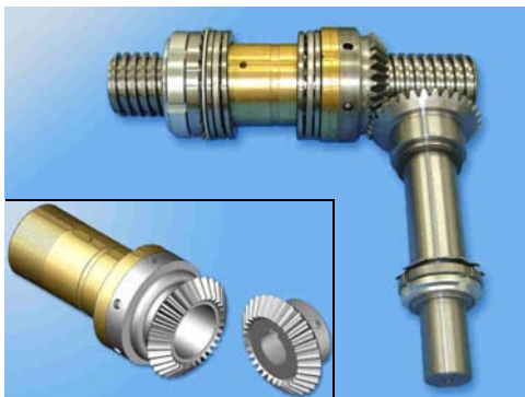
Chiocciola rotante con Coppia conica rapporto 1:1 art.CFB/HR..+CC1:1
